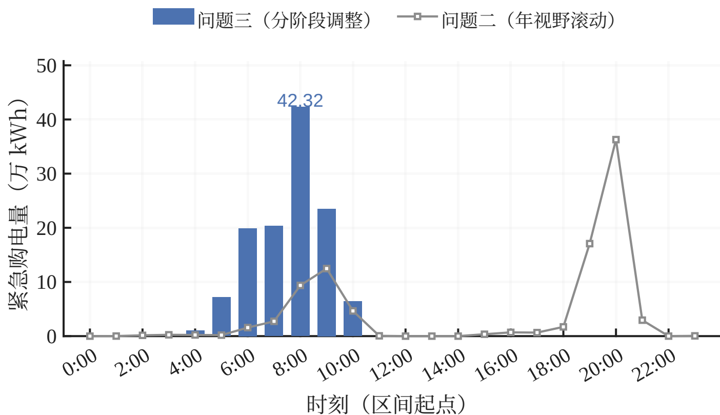
紧急购电的逐时分布：问题三与问题二对照
